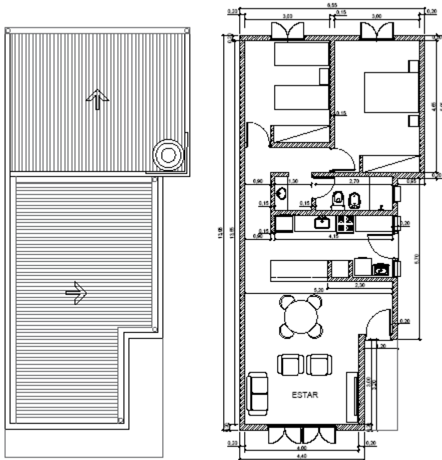
VIVIENDA P.B. -2 D° PLANTA sup. : 78,64 m2
